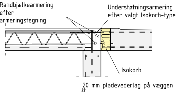
Fastgørelse af altan med termisk beslag
